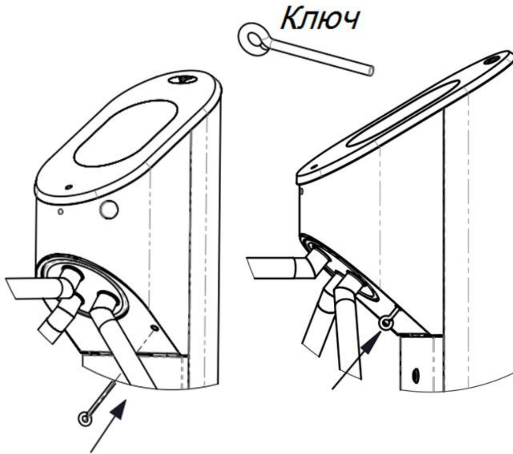
Рисунок 9 – Расположение отверстия на нижней панели для механического складывания панелей.
